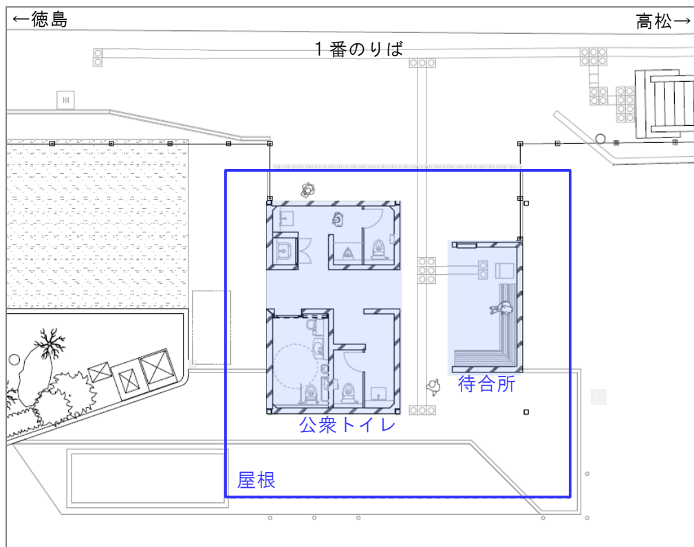
建物平面図
